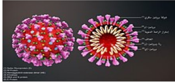
نموذج لمقطع عرضي في فيروس كورونا
